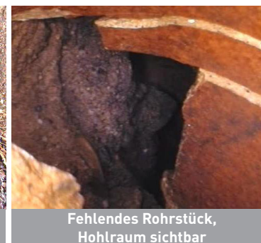
Wurzeinwuchs an undichter Rohrverbindung
