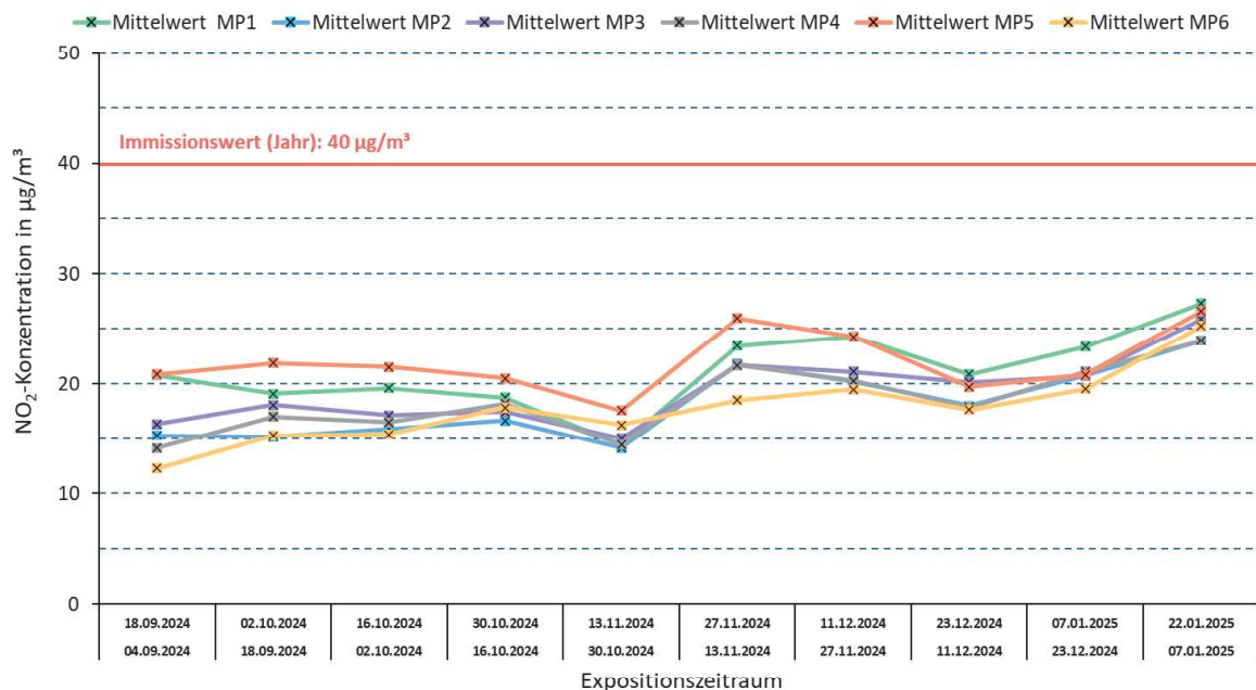
Abbildung 1: Stickstoffdioxidkonzentrationen (ca. 14-tägige Mittelwerte) in Neckarsulm.
